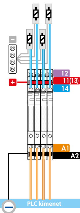
Beavatkozó szervek
