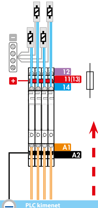
PLC kimenet
