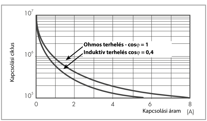
F 40.6 - Villamos élettartam AC terhelésnél
