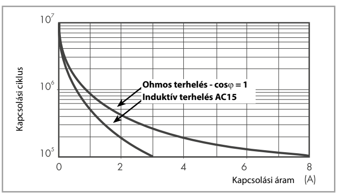
F 40.4 - Villamos élettartam AC terhelésnél
